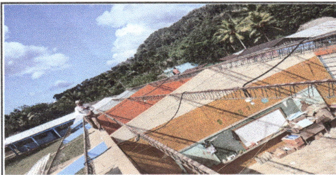
FOTOGRAFIA 3: se observa un avance del 45% en el remozamiento del techo del modulo 2
